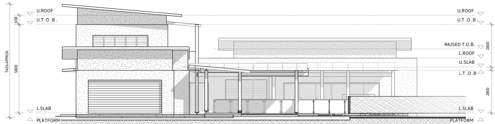
E1 ELEVATION 1 01
