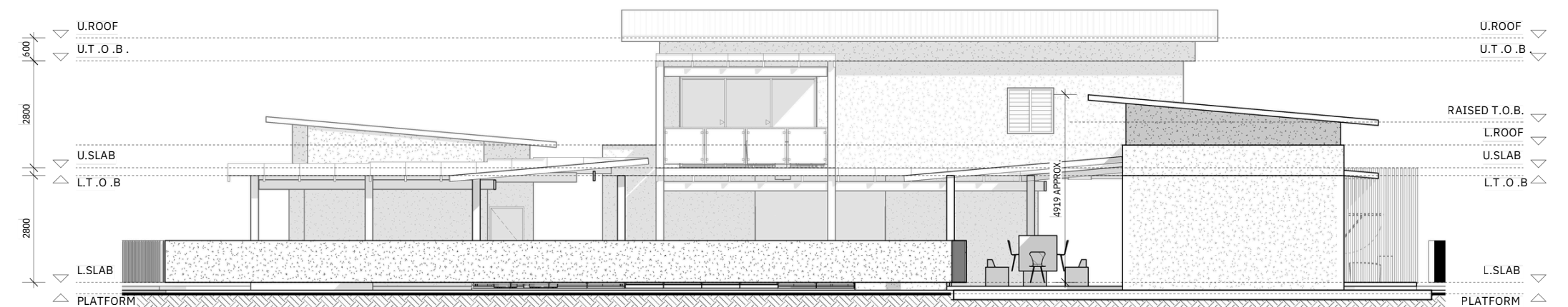
E4 ELEVATION 4 01
