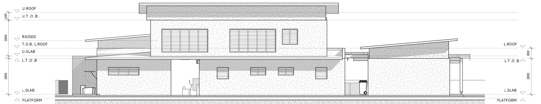
E2 ELEVATION 2 01
